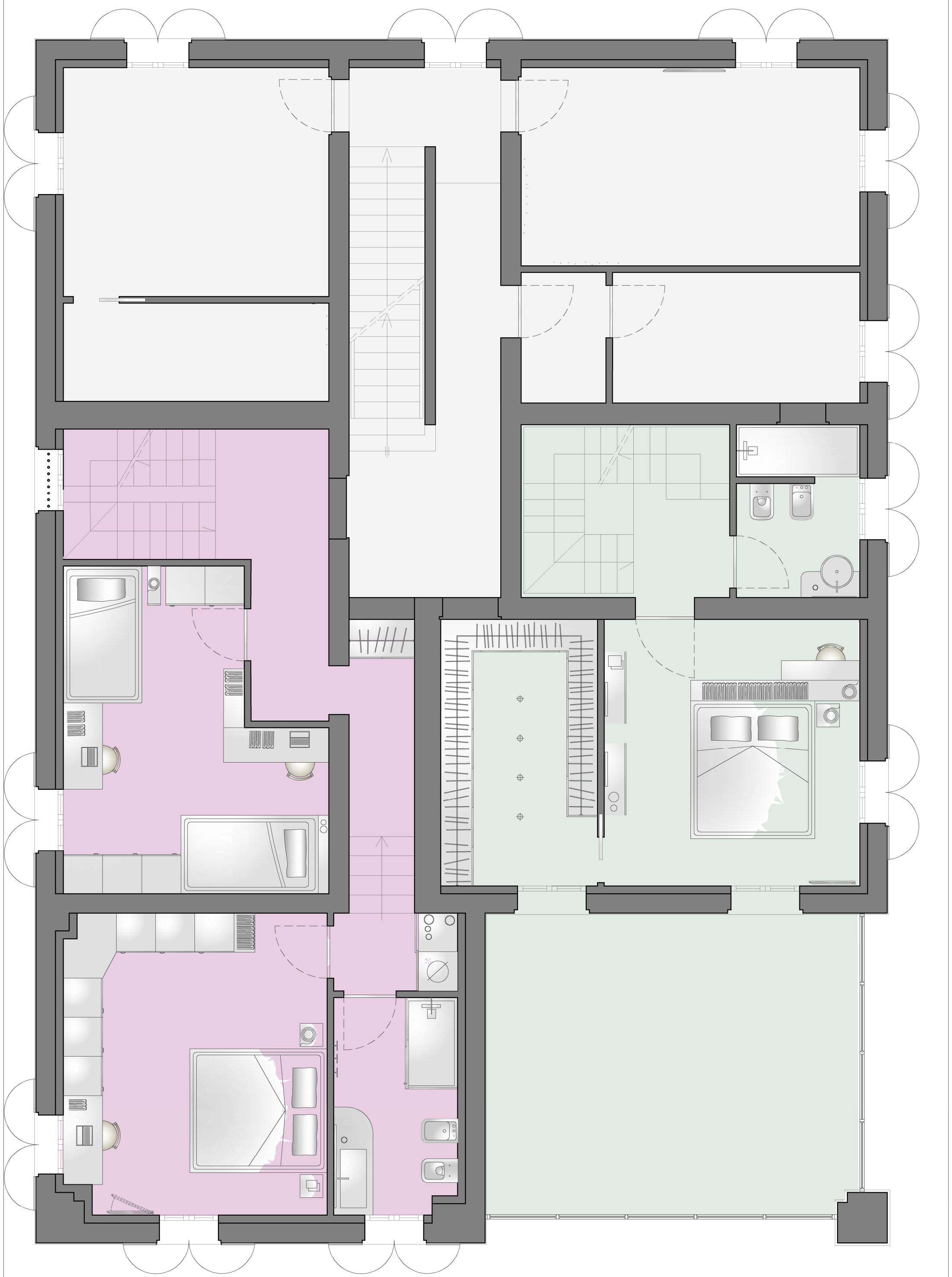
CASA PADRONALE pianta piano primo
