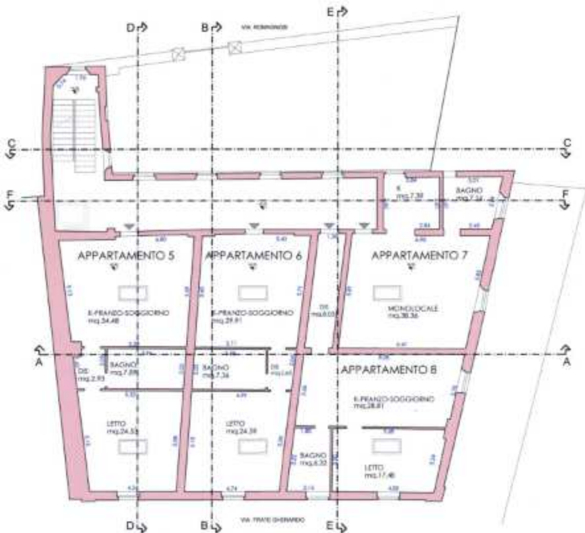
PIANTA PIANO SOTTOTETTO
